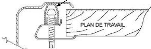
Évier à brides sur rail
