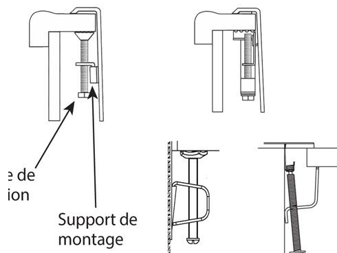
Brides de l'évier
